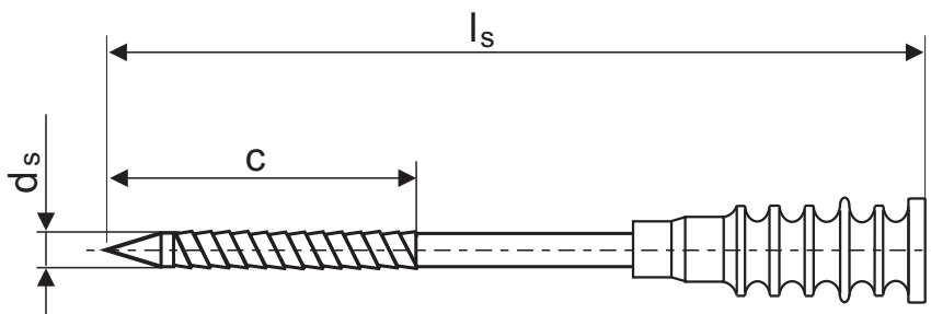
Nagel mit aufgespresstem Kunststoffkopf
